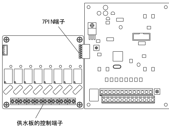
图4 内置供水板连接放大图
