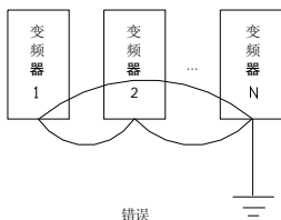
图 2-14 变频器与变频器间接地示意图 2
