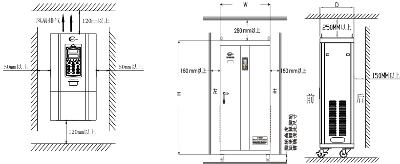
图 2-6(a) 壁挂式变频器安装间隔距离
