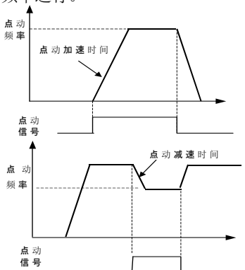
图 5-16 点动运行
