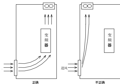
图 2-7 变频器安装环境中通风扇位置
