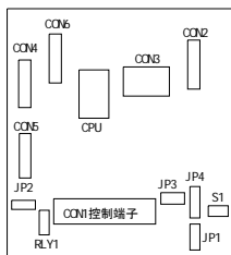
图 2-29(a) P3-3.7 及以下功率的 JP 跳线位置
