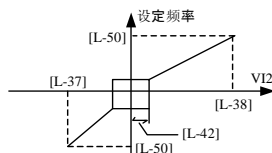
图 5-20 双极性控制 ( [L-41] = 1 ) 时 VI2 与设定频率的对应关系
