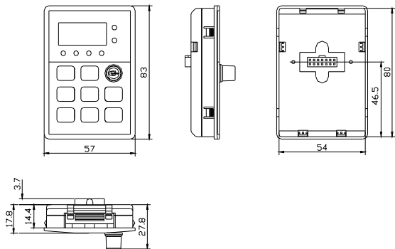
图 2-2 数码显示操作面板尺寸
