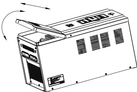
图 2-4 盖板的拆卸和安装
