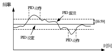
图 5-34 PID 控制允许偏差限值
