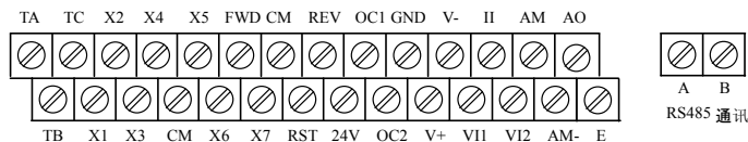
图 2-28 控制回路端子图
