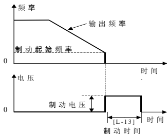
图 5-15 停机时的直流制动功能
