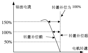
图 5-23 转差频率补偿示意图
