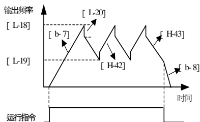
图 5-29 摆频运行（方式 4）
