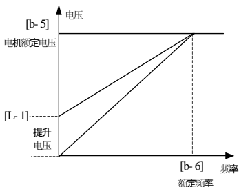
(b) 恒转矩曲线转矩提升示意图
