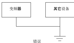
图 2-12 变频器与其它设备接地示意图 3
