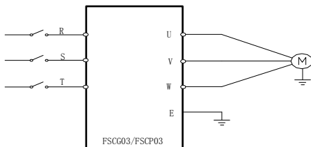
图 2-19 主回路简单配线图
