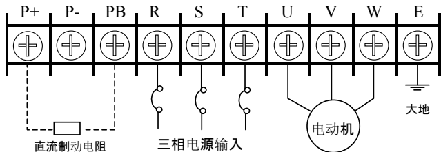
图 2-23 主回路端子台配线图 2
