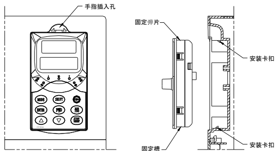
图 2-5 操作面板的拆卸和安装示意图
