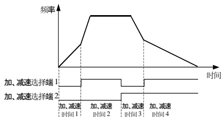
图 5-32 加、减速时间选择
