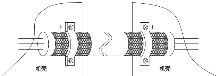
图 2-16 正确的屏蔽接地方法
