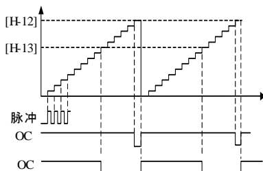
图 5-27 内部计数器功能
