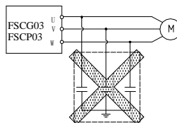
图1-2 变频器输出端禁用电容器示意图
