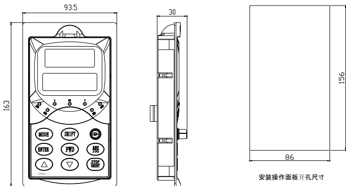
图 2-3 液晶+数码显示操作面板尺寸、安装开孔尺寸
