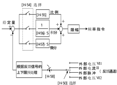
图 5-33 PID 控制器的结构
