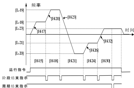
图 5-28 保持最终值模式（方式 3）
