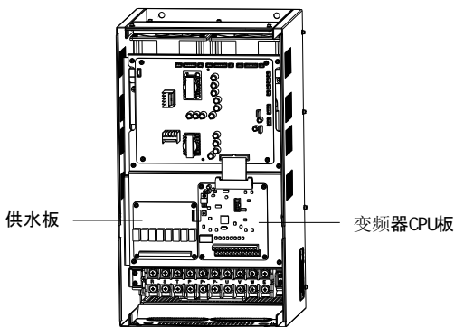
图3 供水附件在变频器内的摆放位置（内置）
