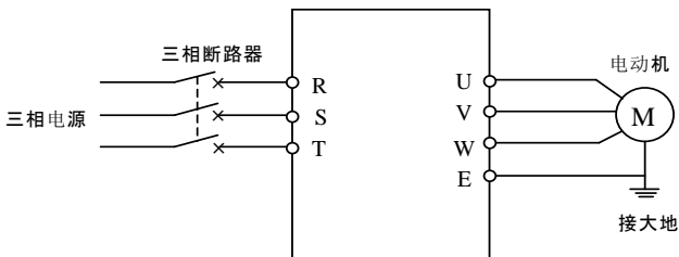
图 3-2 简单运行接线图
