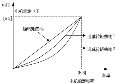
图 5-10 V/F 曲线
