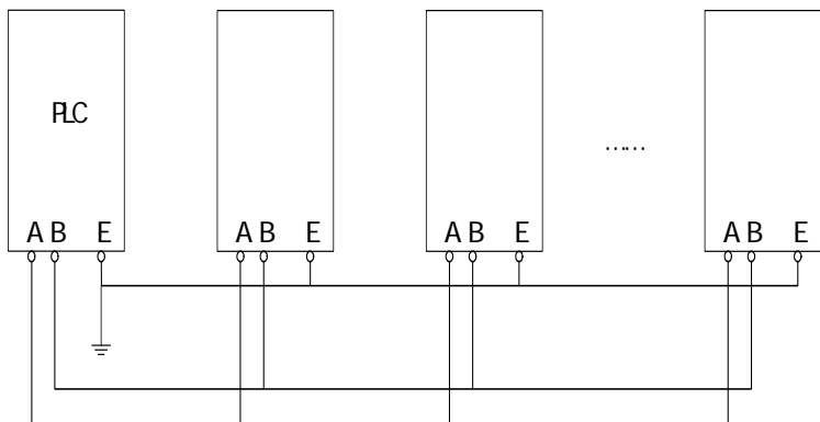
图 2-40 多台变频器在同一 RS485 系统中配线示意图
