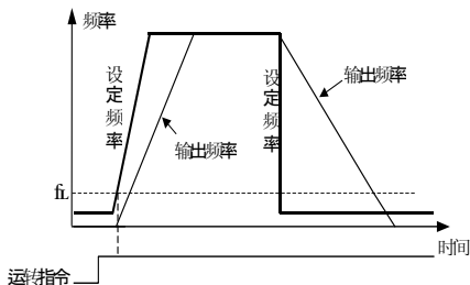
图 5-12 停止模式（[L-5] = 0）时的下限频率作用方式
