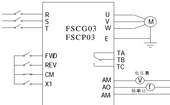
图 7-2 三线制控制模式基本接线图
