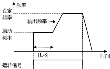
图 5-13 启动频率方式启动
