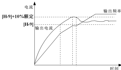
图 5-25 加速中的电流限制功能
