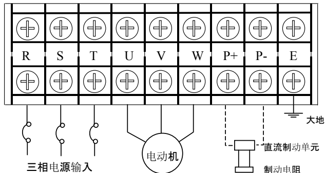
图 2-24 主回路端子台配线图 3
