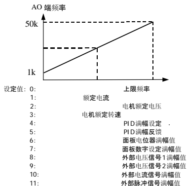
图 5-5 [b-13] = 5.00
