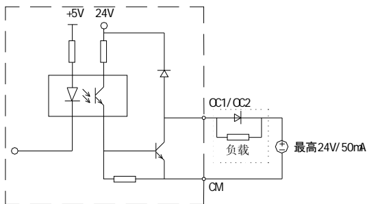
图 2-37 OC1、OC2 输出外部电源方式
