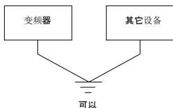
图 2-11 变频器与其它设备接地示意图 2
