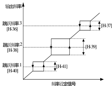
图 5-31 跳跃频率及幅度示意
