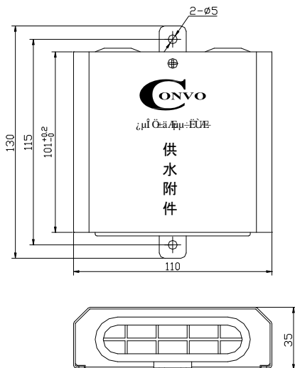
图 1 供水附件外形尺寸
