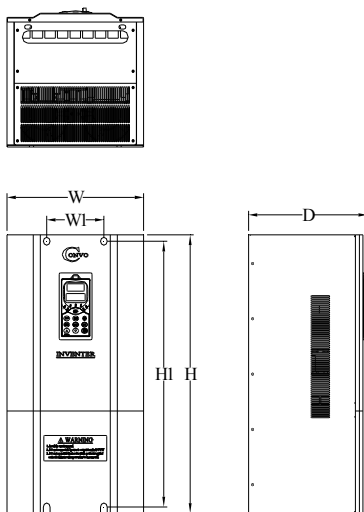
图 2-1 变频器安装示意图
