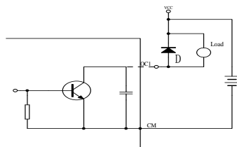
图 5-6 OC 输出端子的内部线路
