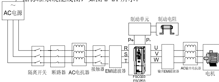
图 2-21 标准系统配线图
