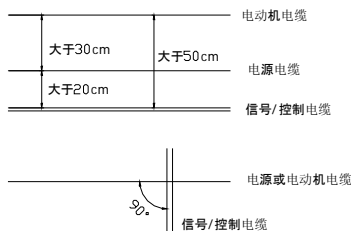
图 2-15 系统配线要求
