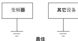
图 2-10 变频器与其它设备接地示意图 1
