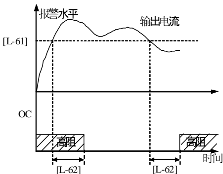
图 5-9 过载报警示意图
