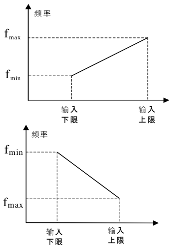
图 5-21 输入量与设定频率的对应关系
