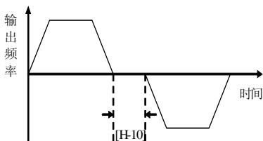
图 5-26 正反转之间的死区
