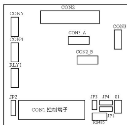
图 2-29(b) G3-3.7 及以上功率的 JP 跳线位置
