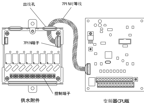
图 2 供水附件与变频器的连接（外置）
