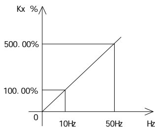
图 5- 22 数字量与增益的对应关系
