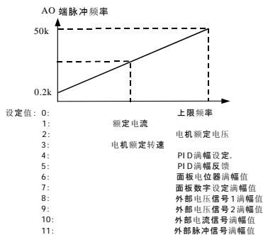
图 5-3 频率输出端子 AO 的输出内容
