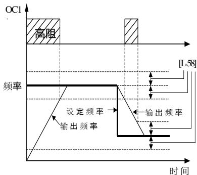
图 5-7 频率到达信号
