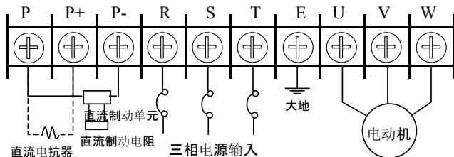
图 2-25 主回路端子台配线图 4
