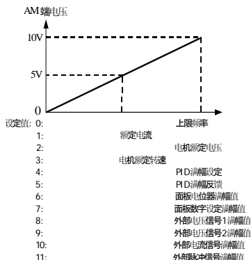
图 5-2 模拟输出端子 AM 的输出内容
