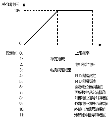
图 5-4 [b-12] = 2.00
