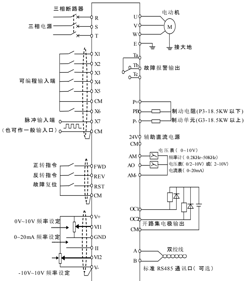
图 2-18 基本运行配线图
