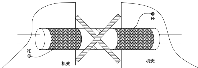
图 2-17 错误的屏蔽接地方法
