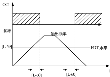
图 5-8 频率水平检测 (FDT)
