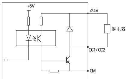
图 2-38 OC1、OC2 输出内部电源方式
