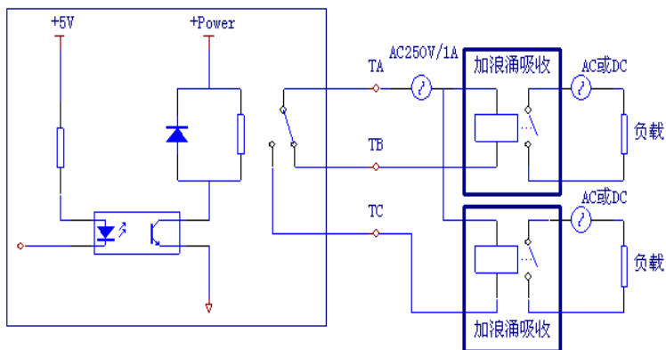
图 2-39 继电器输出端子 TA、TB、TC 配线图
