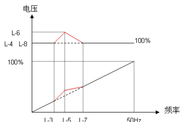
图 5-4 (b) V/F 曲线修正
