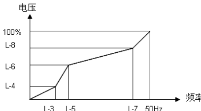
图 5-4 (a) 自定义 V/F 曲线设定
