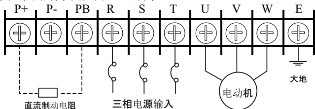
图 2-24 主回路端子台配线图 3
