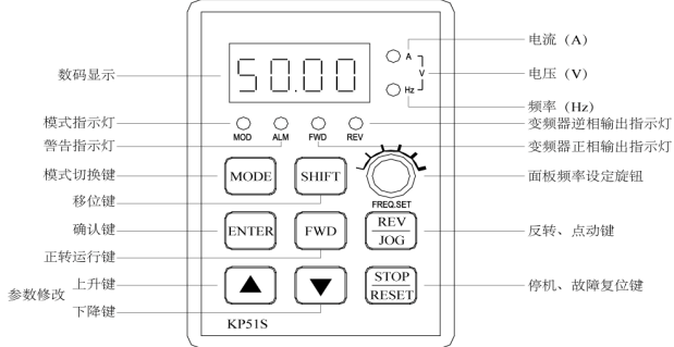
图 3-1 操作面板布局图 1
