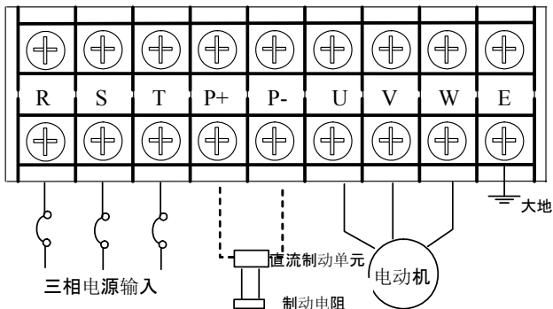
图 2-25 主回路端子台配线图 4
