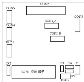
图 2-31 (b) G5-11KW 以上 JP 跳线位置
