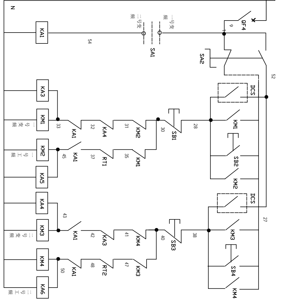
一拖二变频控制电路图
