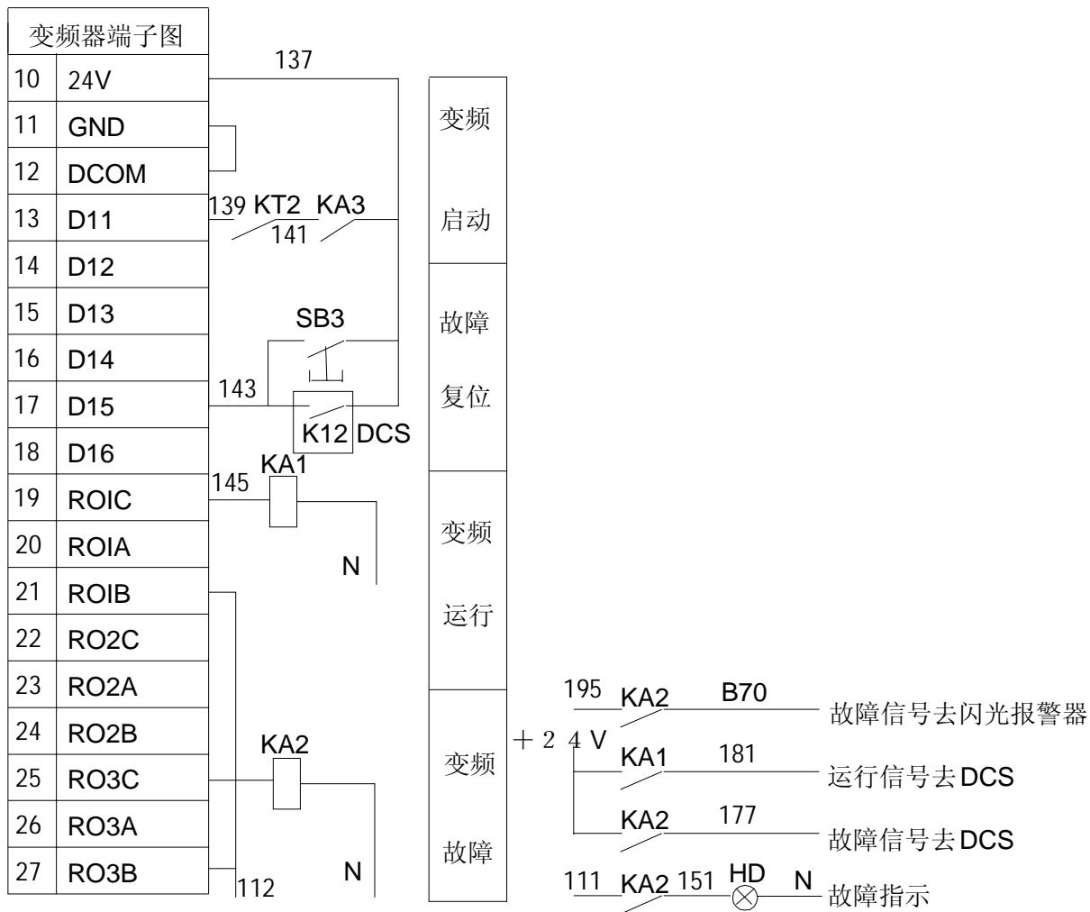
引风变频器端子接线图
